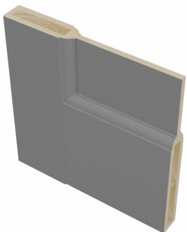
Разрез полотна серии ТУРИН Neo, филенка 10мм. Царга 125x38мм.
